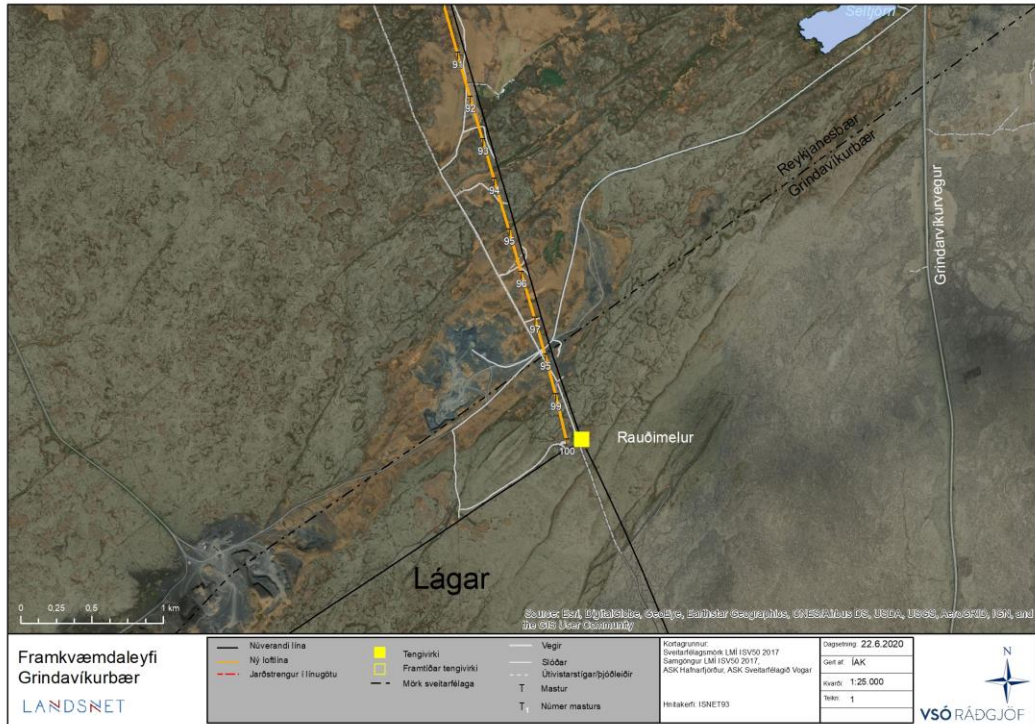
Mynd 3.1: Yfirlitsmynd af línuleið Suðurnesjalínu 2 í Grindavík
